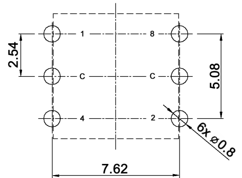
P.C.B. DIMENSION
